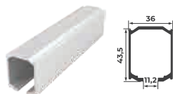
7 Верхняя направляющая
